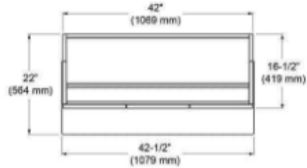
201 Plan
