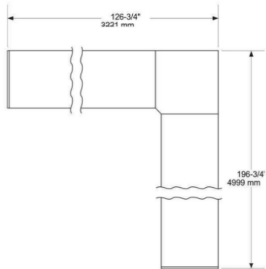
594 Plan
