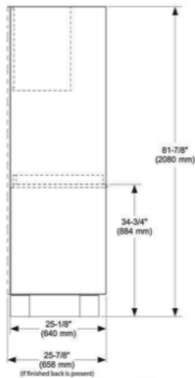
594 Elevation - Side
