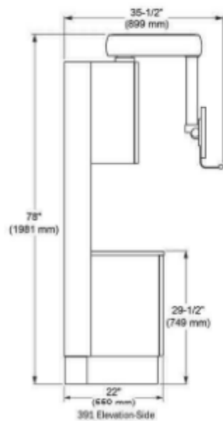
391 Elevation Side
